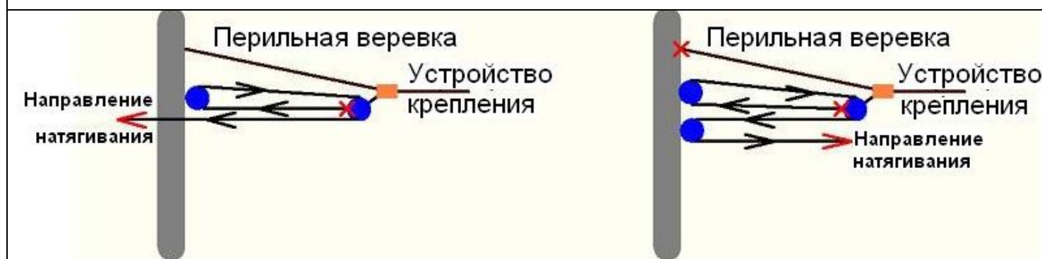
«Полуторный полиспаст» (3:1)
