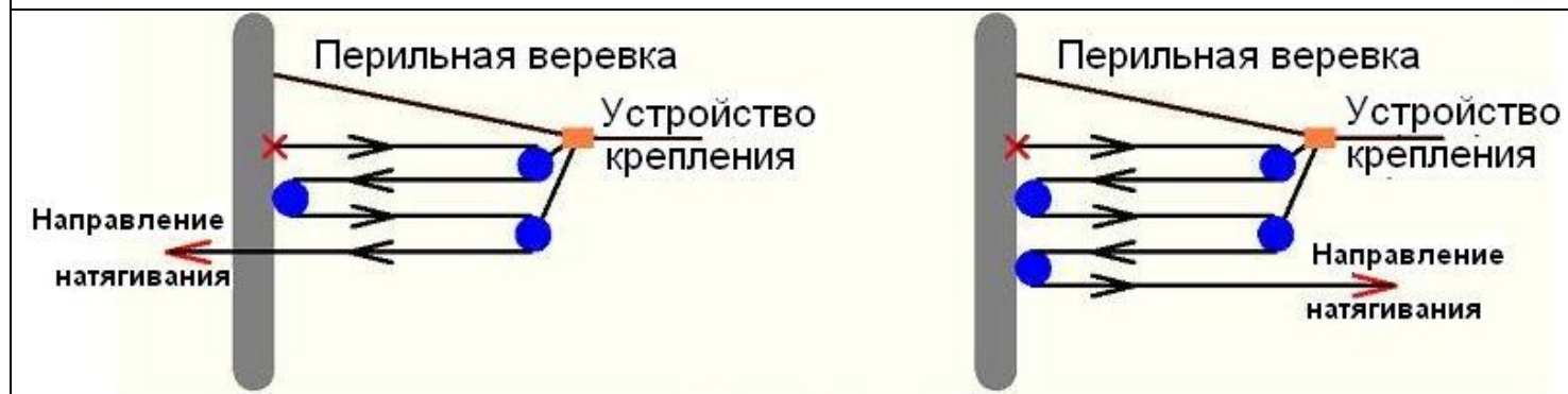
«Двойной полиспаст» (4:1)
